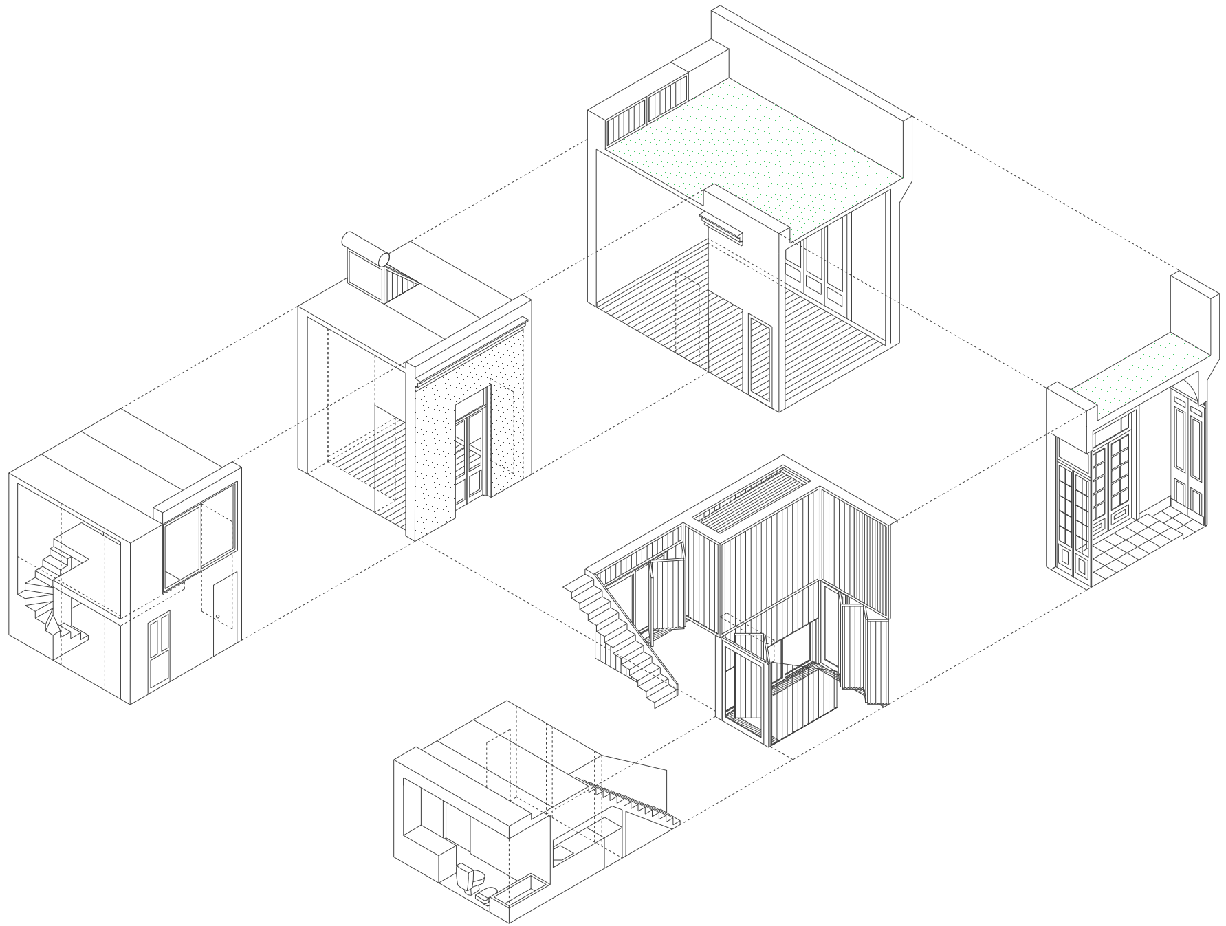
AXONOMÉTRICA DESPIEZADA
