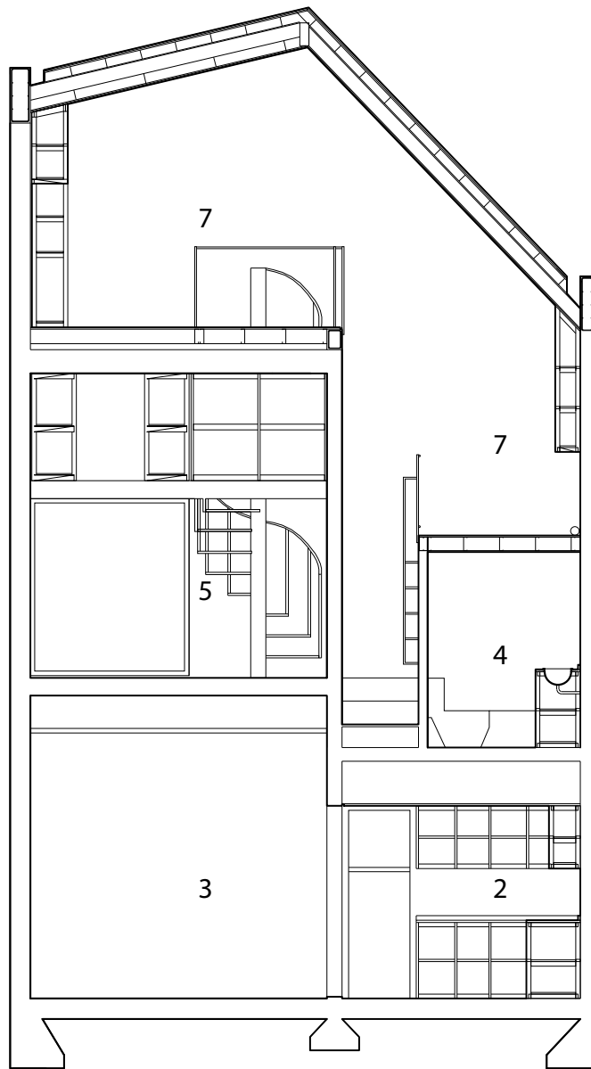
CORTE DD
