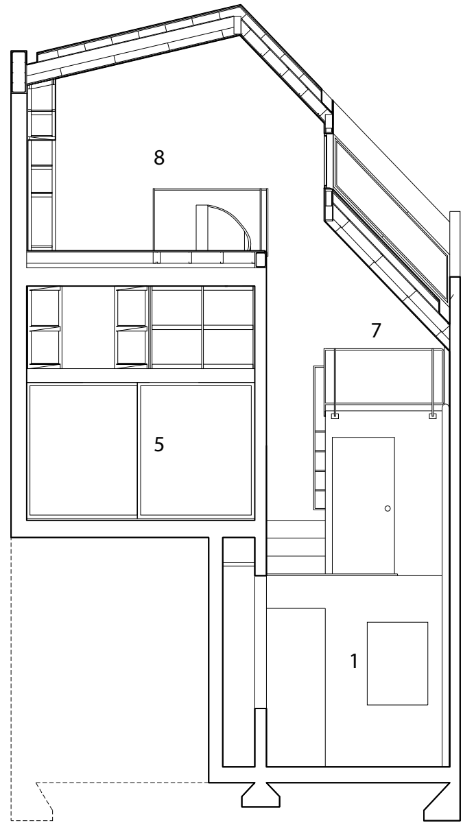
CORTE CC
