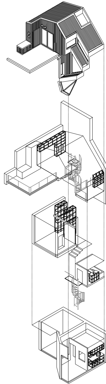
AXONOMÉTRICA DESPIEZADA
