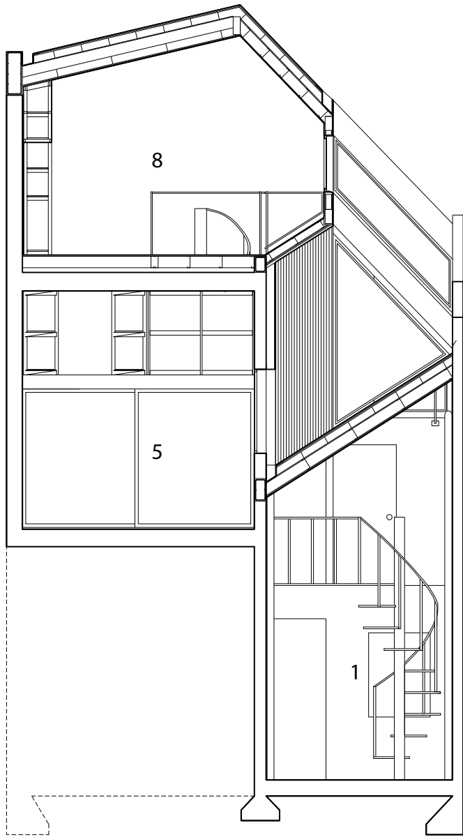
CORTE BB
