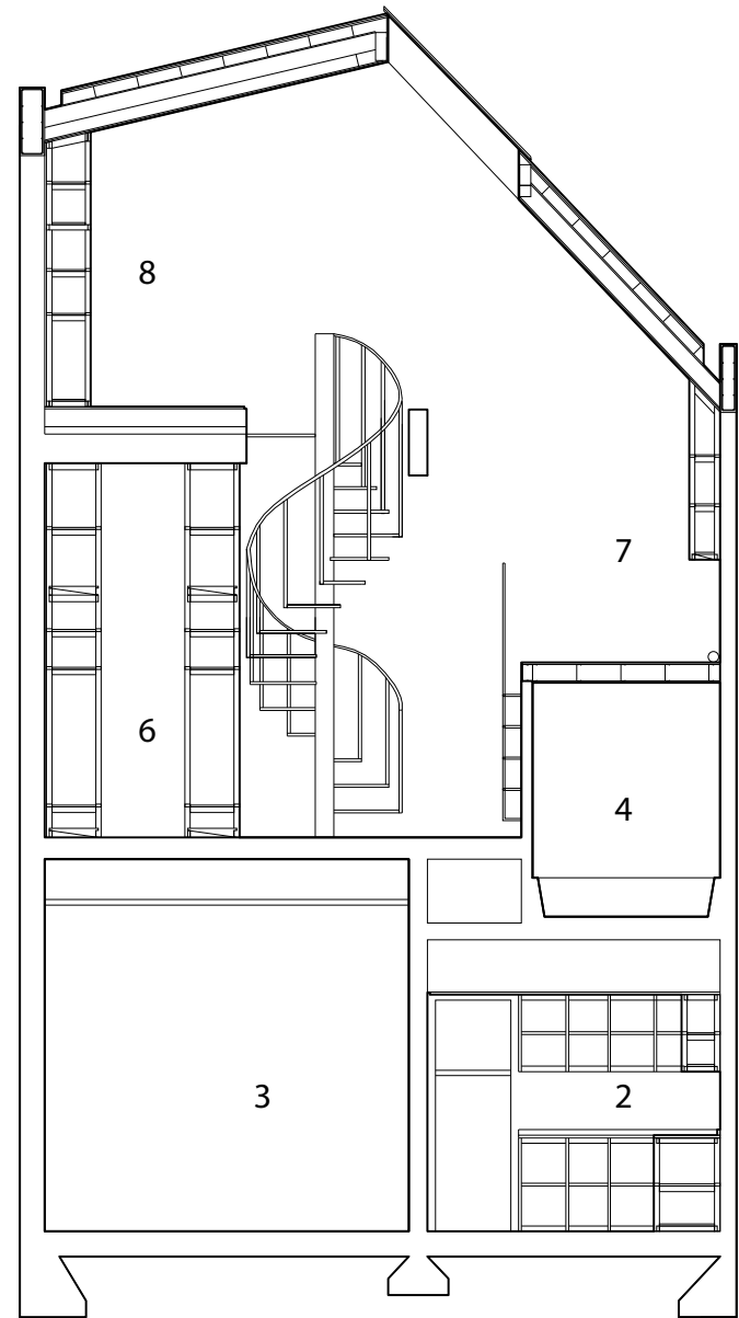
CORTE EE
