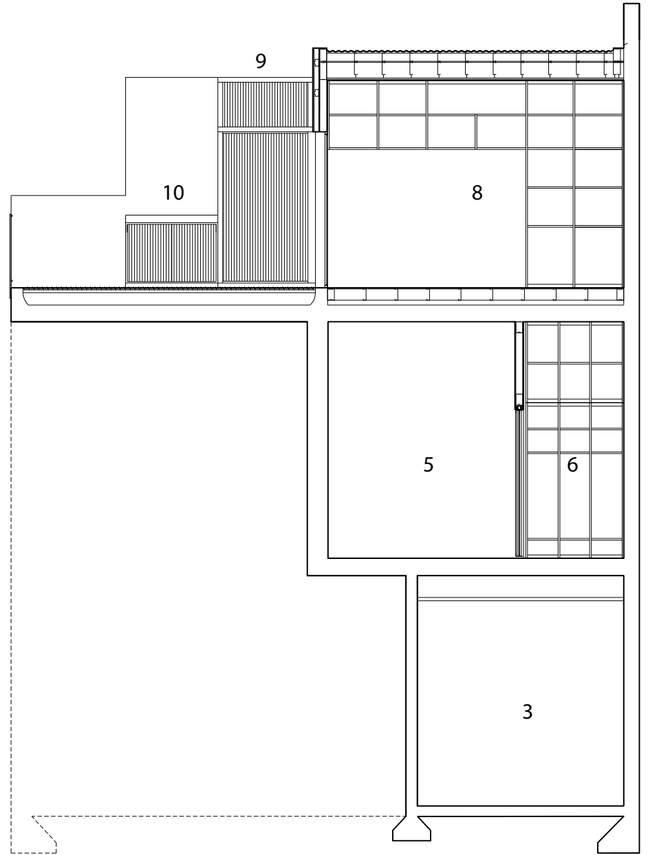
CORTE HH
